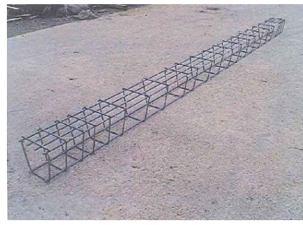
消雪用ブロック用の鉄筋かご
